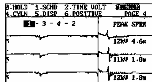
Рис. 4-9. Смещение модели системы зажигания
