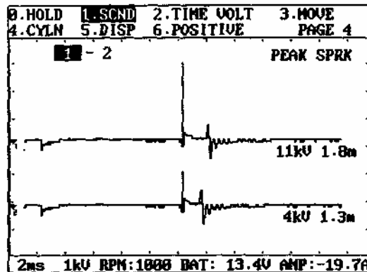
Рис. 4-30. Вторичная модель – DLI катушка с двумя выходами
